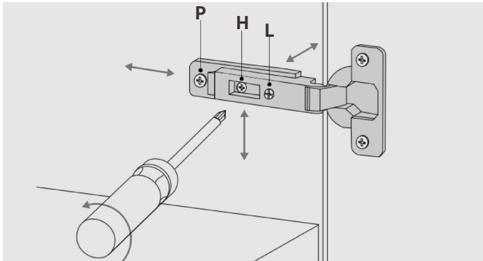
P - Einstellung Türtiefe H - Einstellung Türhöhe L - Einstellung Türbreite
