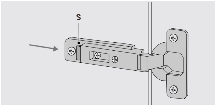
S - Türschnellspannhebel
